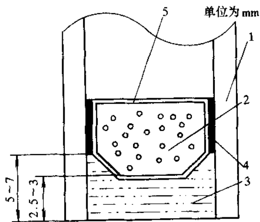
图1 密封胶厚度
