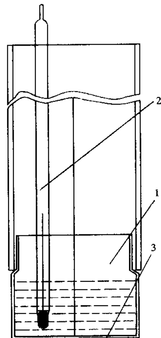
图5 露点仪
