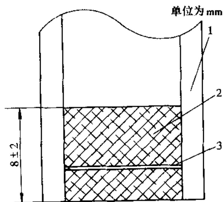
图2 胶条厚度
