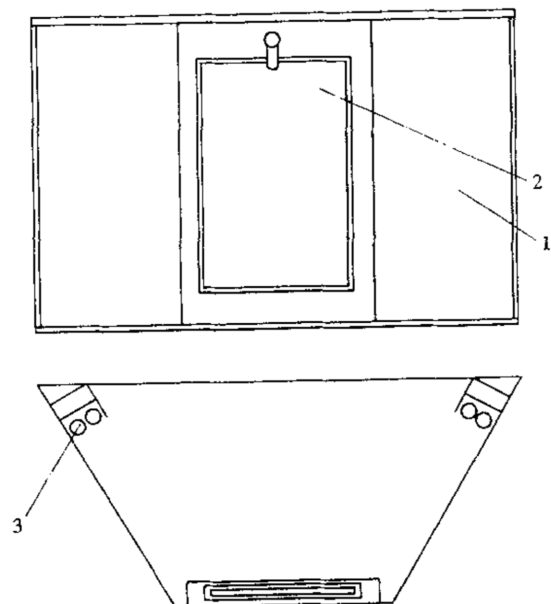
图3 观察箱
