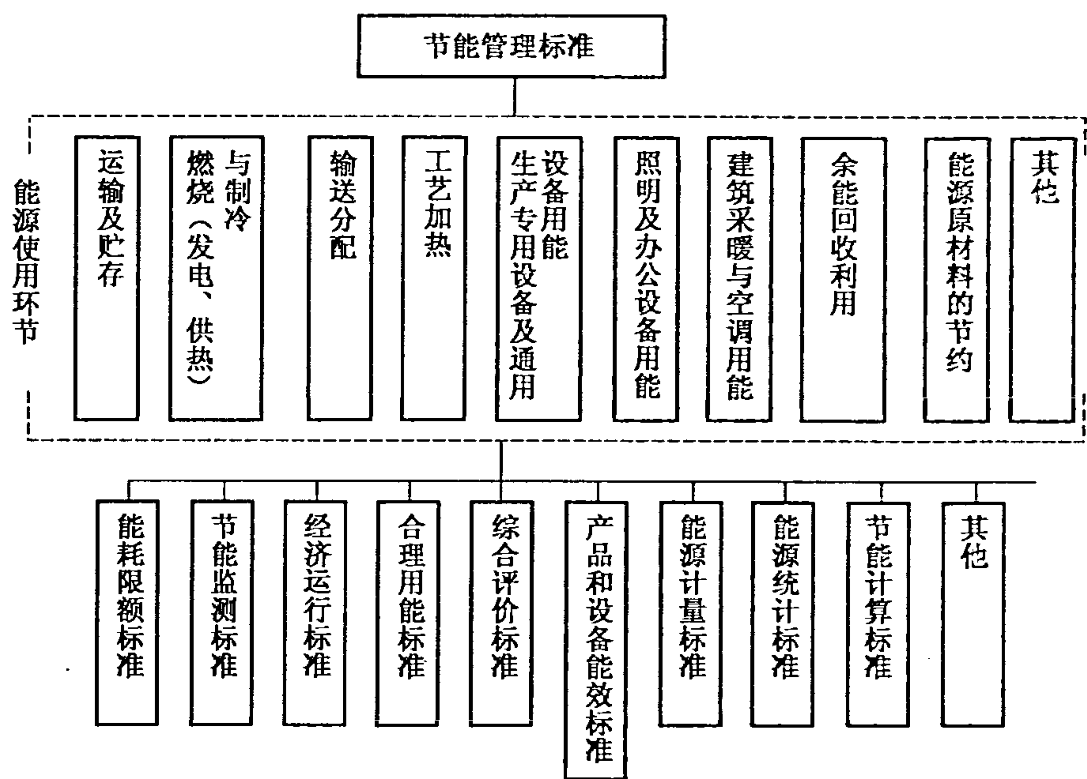
图 4 节能管理标准子体系的结构层次图
